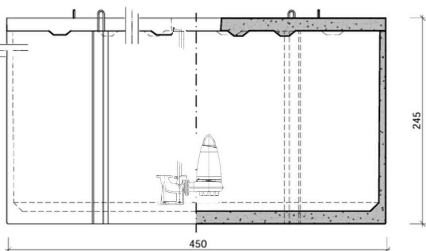
VOORAANZICHT / DOORSNEDE VUE FRONTALE / COUPE
